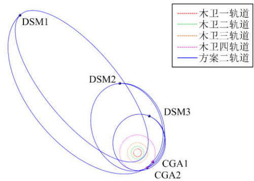
图 2 方案二木星系内转移轨道
