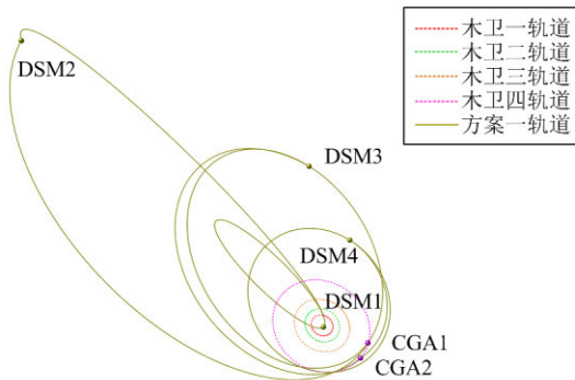
图 1 方案一木星系内转移轨道
